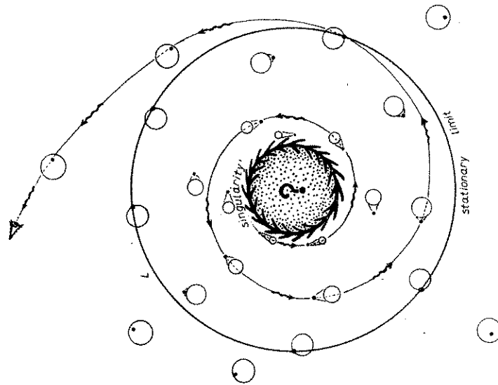
Fig. 6. — A « naked singularity » (Kerr-Newman solution with m^2 < a^2 + e^2 ).
